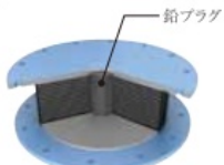
ゴムアイソレータ イメージイラスト
