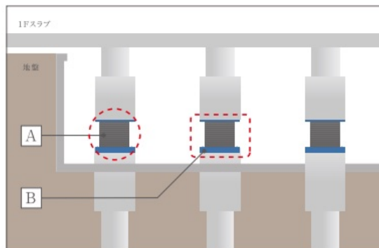
免震装置概念図
