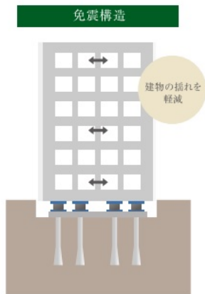
免震部材が地震の振動を吸収し、平行にゆっくりとした揺れに変わる。
